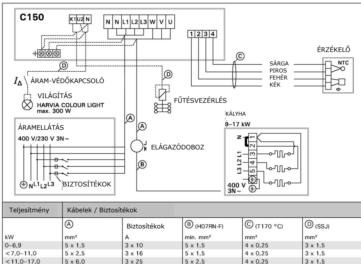
10. ábra: A C150 vezérlőegység és a HL kályha elektromos csatlakozásai
