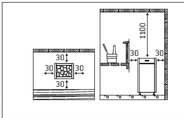
4. ábra: Minimális biztonsági távolságok (minden méret milliméterben megadva)
