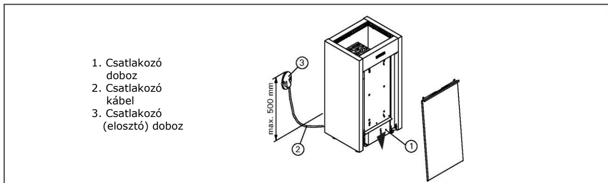
7. ábra: A kályha csatlakozásai
