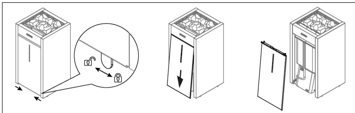
5. ábra: A szervizborítólappal kinyitása
