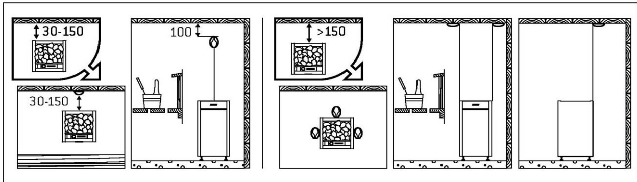
6. ábra: A hőmérsékletérzékelő beszerelése (minden méret milliméterben megadva)
