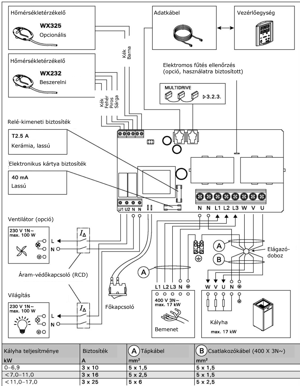
11. ábra: A C150 vezérlőegység és a HL kályha elektromos csatlakozásai
