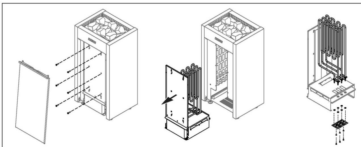
8. ábra: A fűtőelemek cseréje
