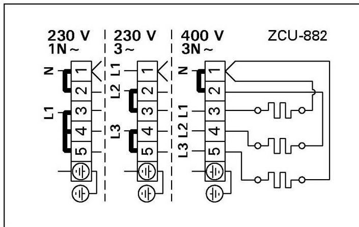
9. ábra: Elektromos csatlakozások
